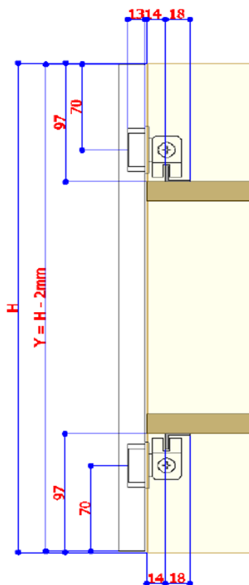
MONTAJE CON GUIA EN LA PARTE EXTERIOR DEL MUEBLE
