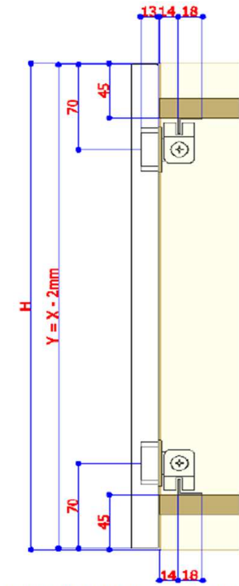
MONTAJE CON GUIA EN LA PARTE INTERIOR DEL MUEBLE
