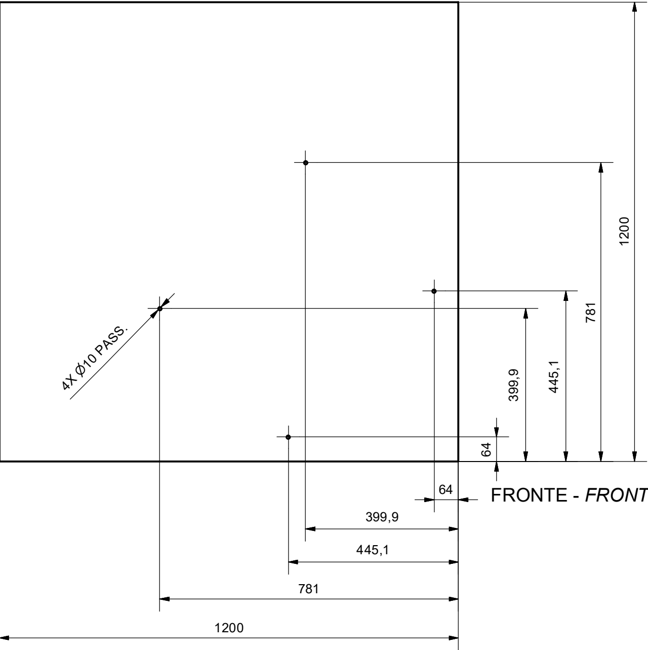
VISTA DALL'ALTO - TOP VIEW
