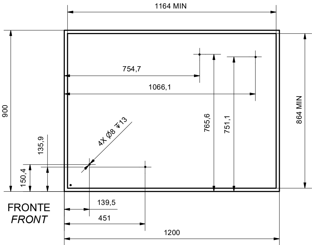
C. Bussola M6 - M6 bush (x 4) VISTA DAL BASSO - BOTTOM VIEW
