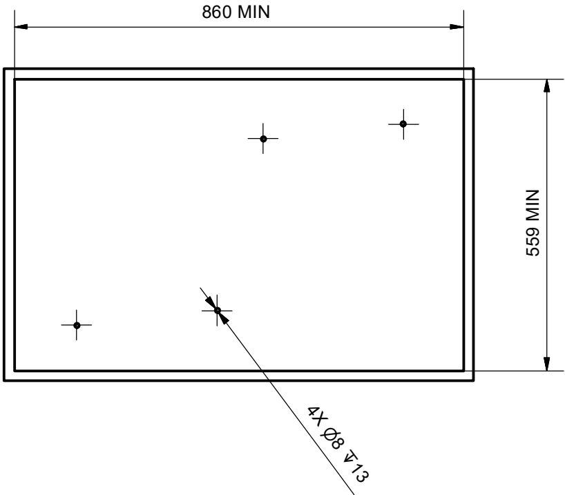
VISTA DAL BASSO - BOTTOM VIEW
