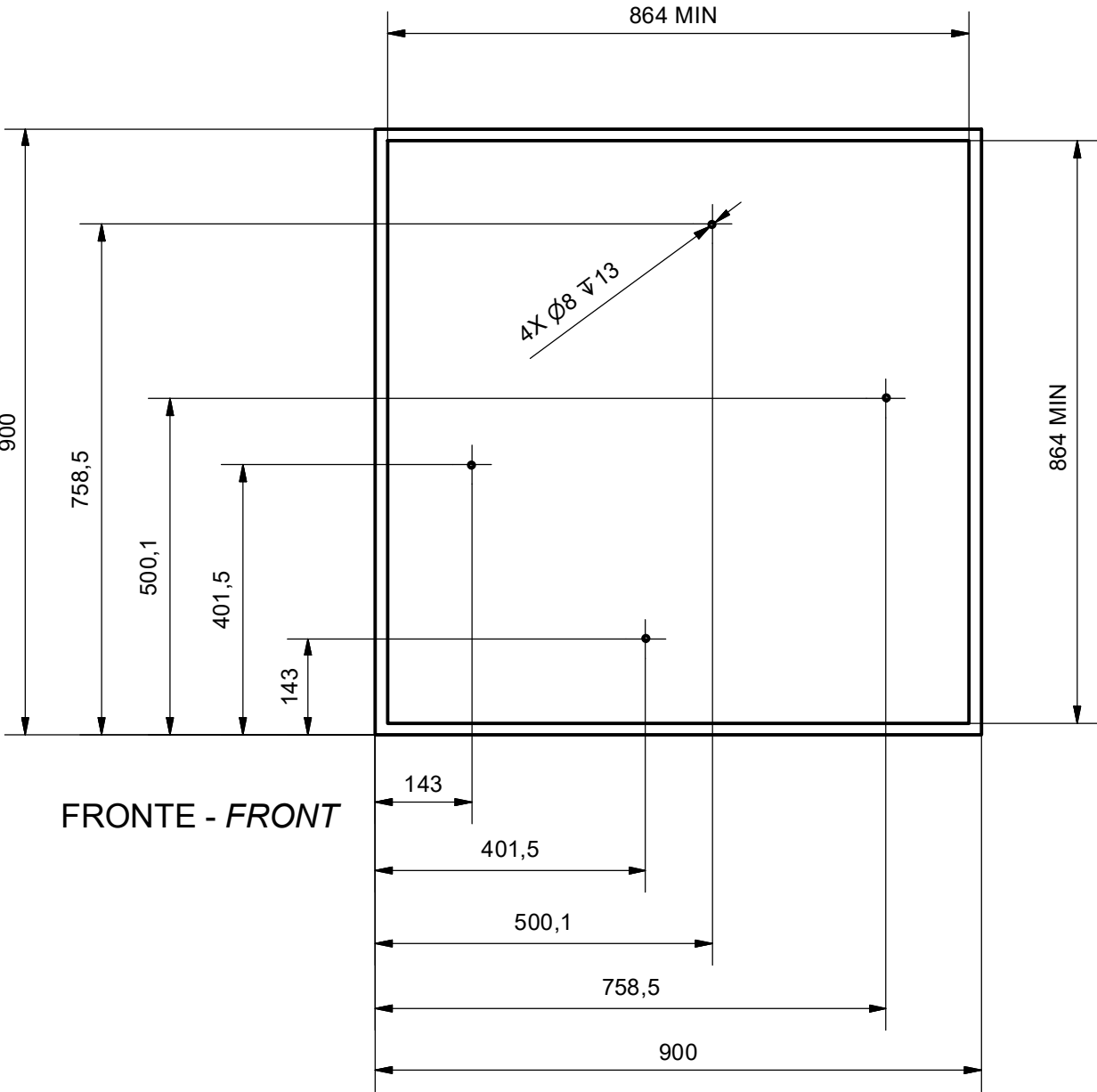
VISTA DAL BASSO - BOTTOM VIEW
