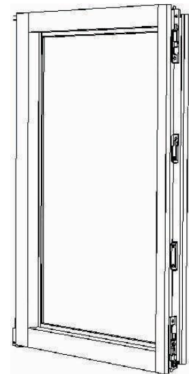
5 - Colocacion pasadores y cerraderos a la hoja.
