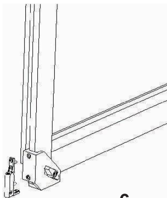
6 - Taladrado y colocacion pernio angular en el marco.
