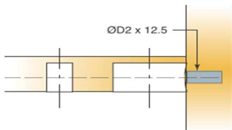
D2= Ø8mm
