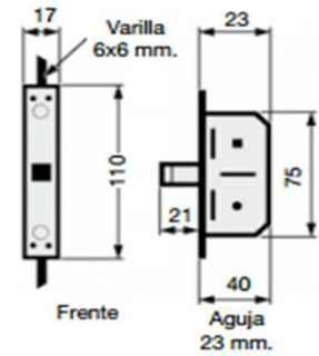
Grisans 3 cierres Cerradero arriba, abajo y en el centro
