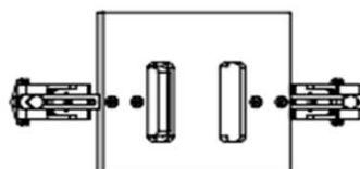
Plantilla para fresado cerraderos en ventanas 2 hojas
