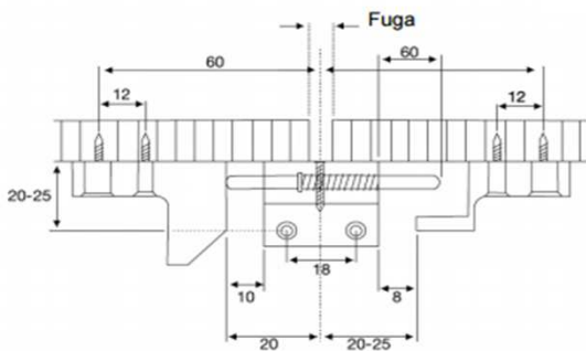
Posición abierto.
