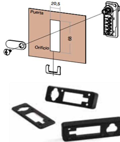
Placas de fijación de diferentes gruesos en función del grueso de la puerta. Incluidas en los kits cerradura.
