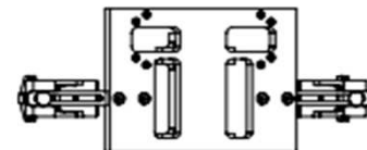
Plantilla para fresado cerraderos
