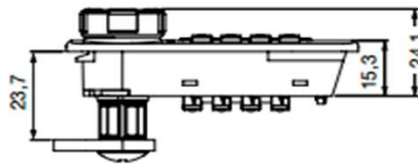
Cerradero
