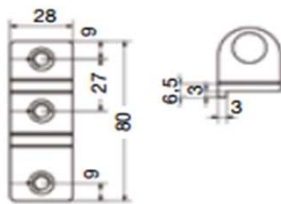
Cerradero
