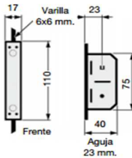
Grisans 2 cierres Cerradero arriba y abajo.
