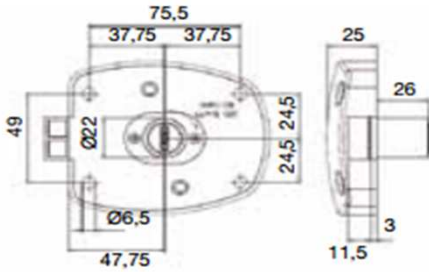
Cerradero
