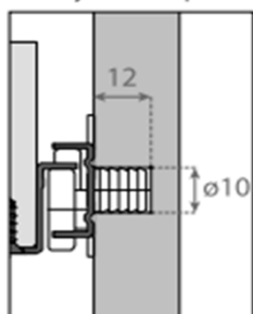
Montaje con casquillos
