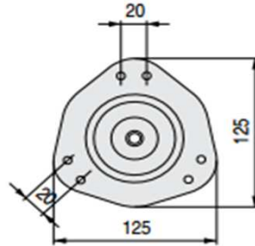
Soporte en hierro acabado zincado
