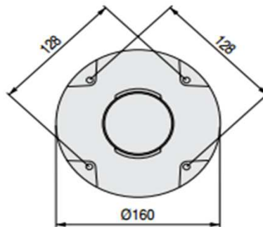
Soporte en plástico acabado negro
