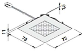
Foco cuadrado Q68
