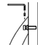
Fijación Simple oculta
